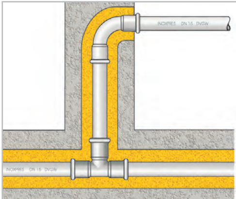
Figura 50a – Creazione di spazi di dilatazione
