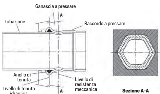
Figura 4 - Vista in sezione di un accoppiamento inoxPRES / steelPRES / aesPRES / marinePRES con ganascia. Nelle dimensioni \varnothing 12 \div 35 mm si ottiene una pressatura esagonale
