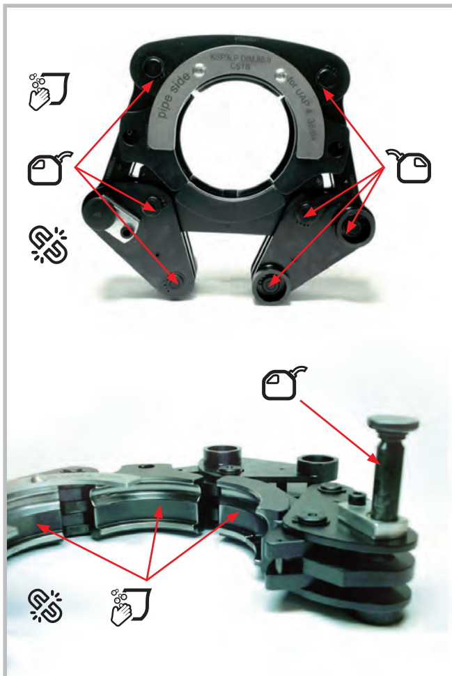
Figura 19 – Attrezzatura Klauke
