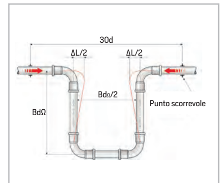
Figura 53 – Compensazione della dilatazione ad U (BdΩ = Bd / 1,8)
